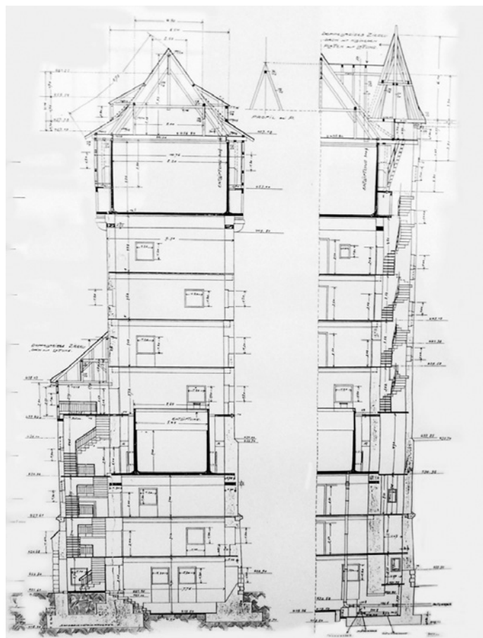
Nach Plänen des Architekten Jürgen Sievers wurde der Wasserturm gebaut. Die handgezeichneten Originale sind noch in der Plankammer vorhanden.
